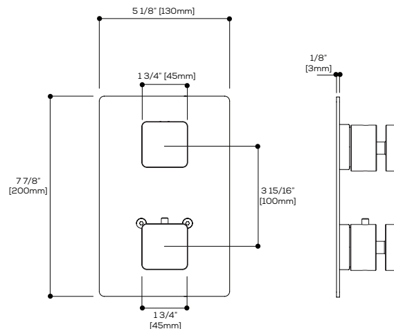
Handle option 2 / Poignée option 2
