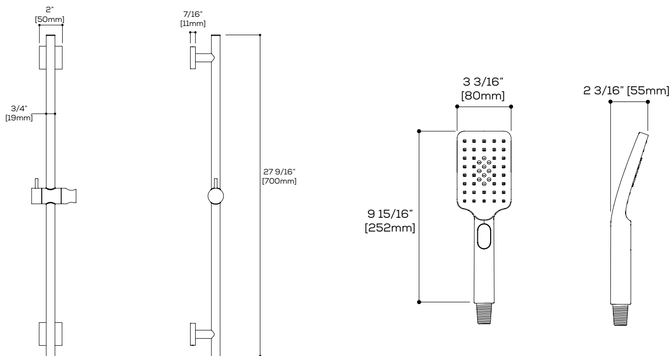
ABSPXPR80 Slider / Curseur
